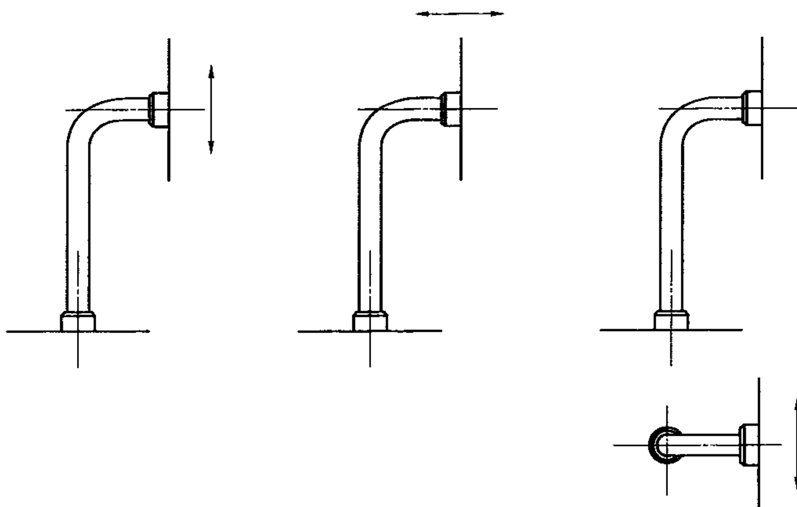
图 C.1 试样的振动方向
